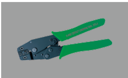
■ 1530 電腦端子壓著鉗 ■ D-SUB CONTACT CRIMPING TOOL KTC-4 適用裸端子: 0.1-0.25 mm 2 / 0.5-1.0 mm 2
