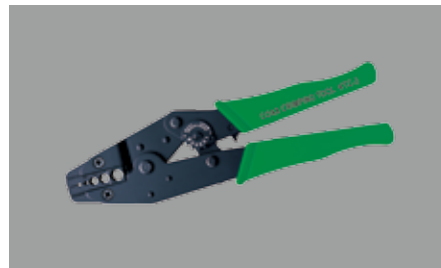
■ 1530 強力電腦接頭壓著鉗 ■ COAX CRIMPING TOOL KTC-3 適用裸端子: 1.72 mm 2 / 2.5 mm 2 / 5.4 mm 2 / 6.48 mm 2 / 8.2 mm 2
