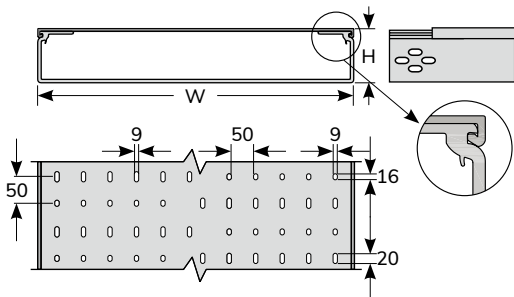
SDH-300100J, 400100, 500100J, 600100
