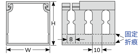
出線孔尺寸
